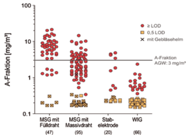
Abbildung 2: Alveolengängiger Schweißrauch (A) nach Schweißverfahren und Nutzung von Gebläsehelmen (Arbeitsplatzgrenzwert 3 \text{ mg/m}^3 )
