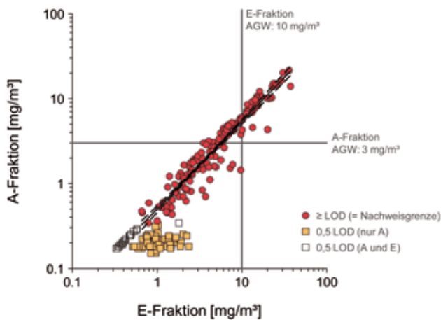
Abbildung 1: Assoziation der Konzentrationen der A- und E-Fraktion des Schweißrauchs auf Probenträgern des Typs 575 (PGP-EA)
